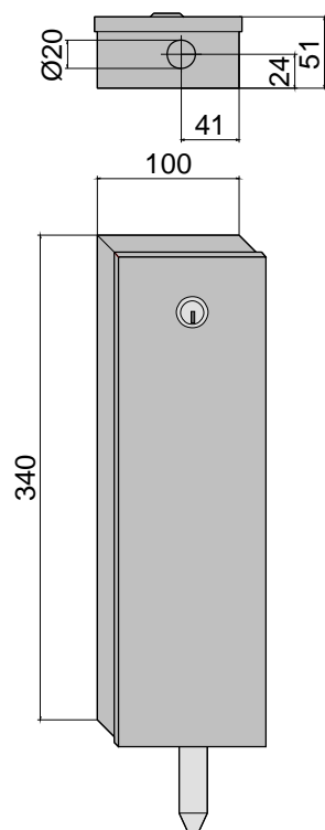
Hauptabmessungen
